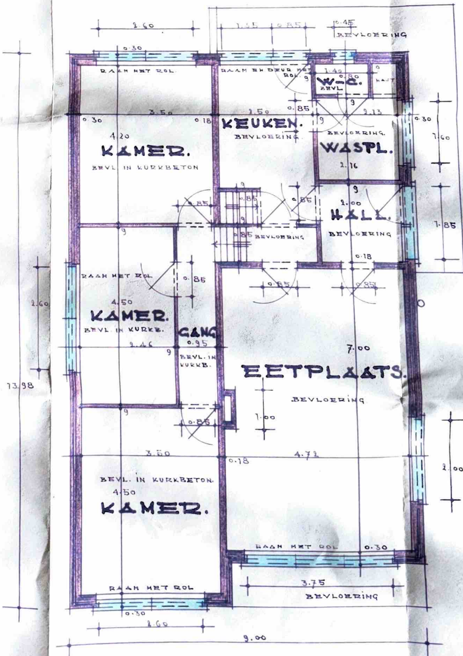
VERDIEPING - GELYKVLOERS.
