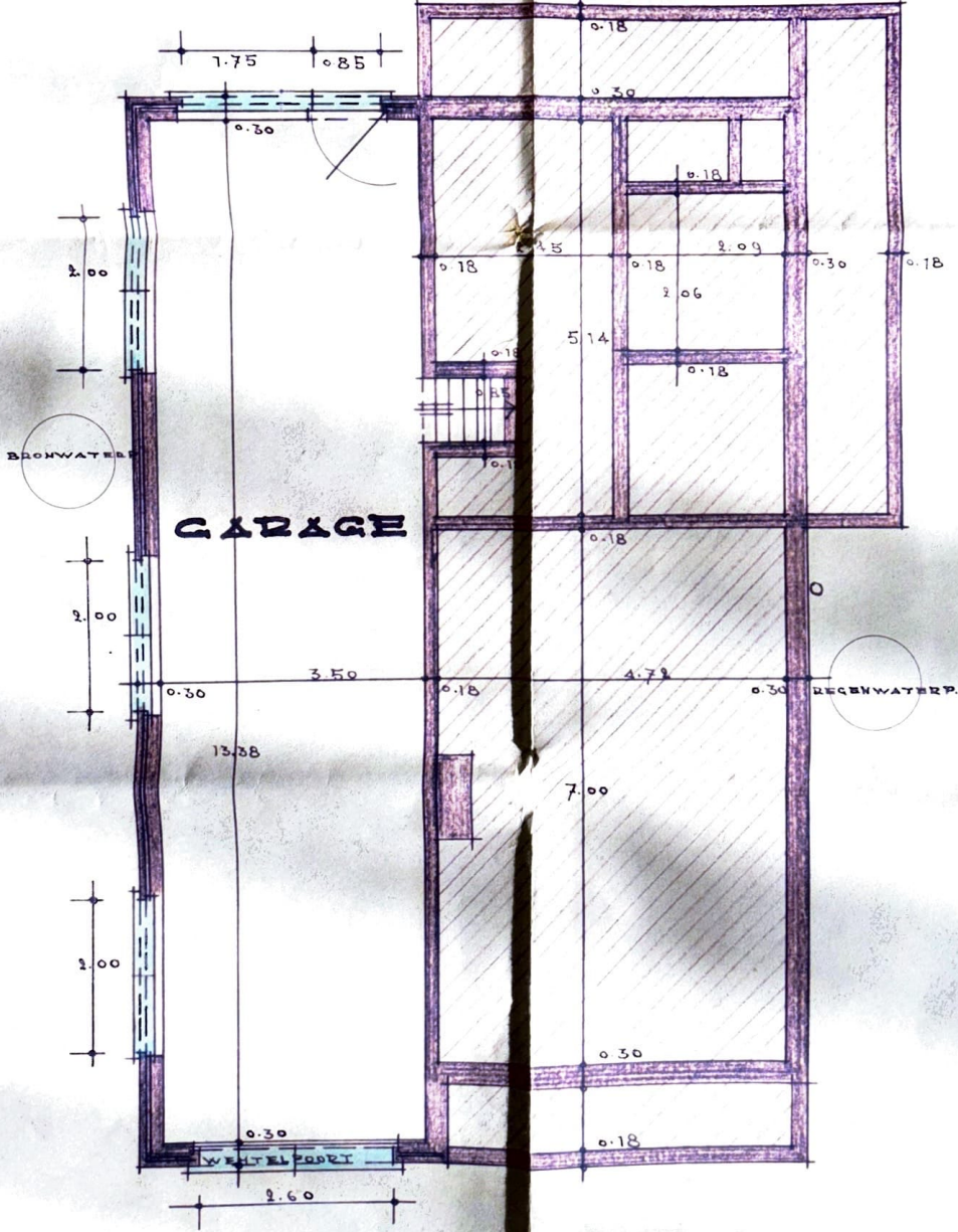
GELYKVLOERS - FUNDERINGEN.
