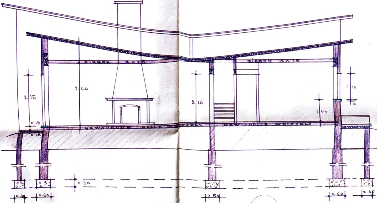
DOORSNEDE.
