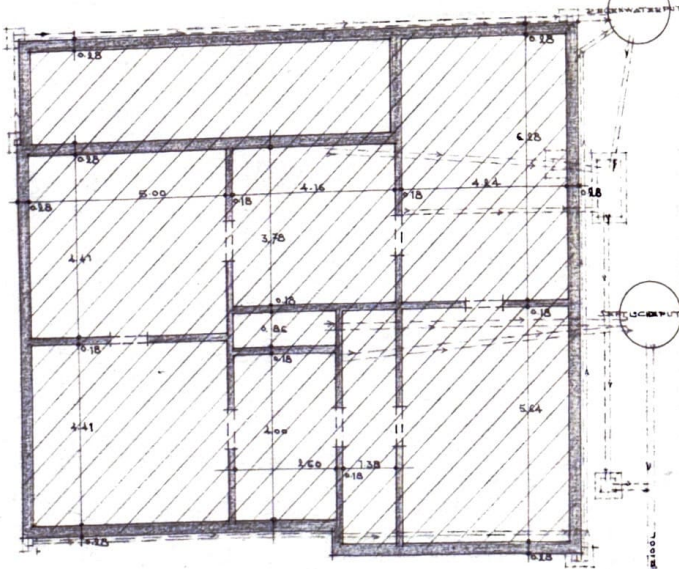
FUNDEERINGEN.
