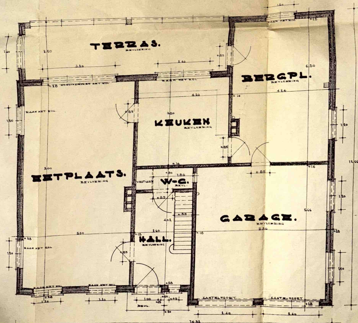
GELYKVLOERS.
