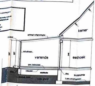
DOORSNEDE AA
