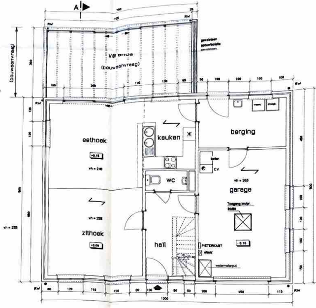
GELIJKVLOERS
