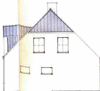
ZIJGEVEL RECHTS
