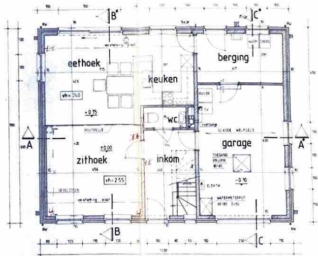
GELIJKVLOERS
