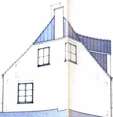
ZIJGEVEL LINKS
