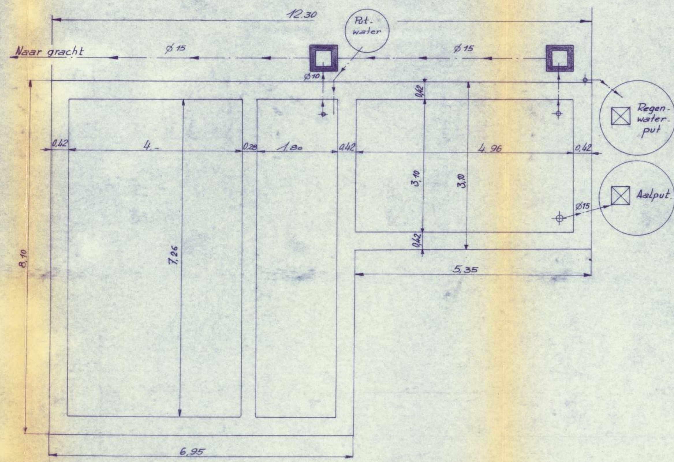
FUNDERINGEN.
