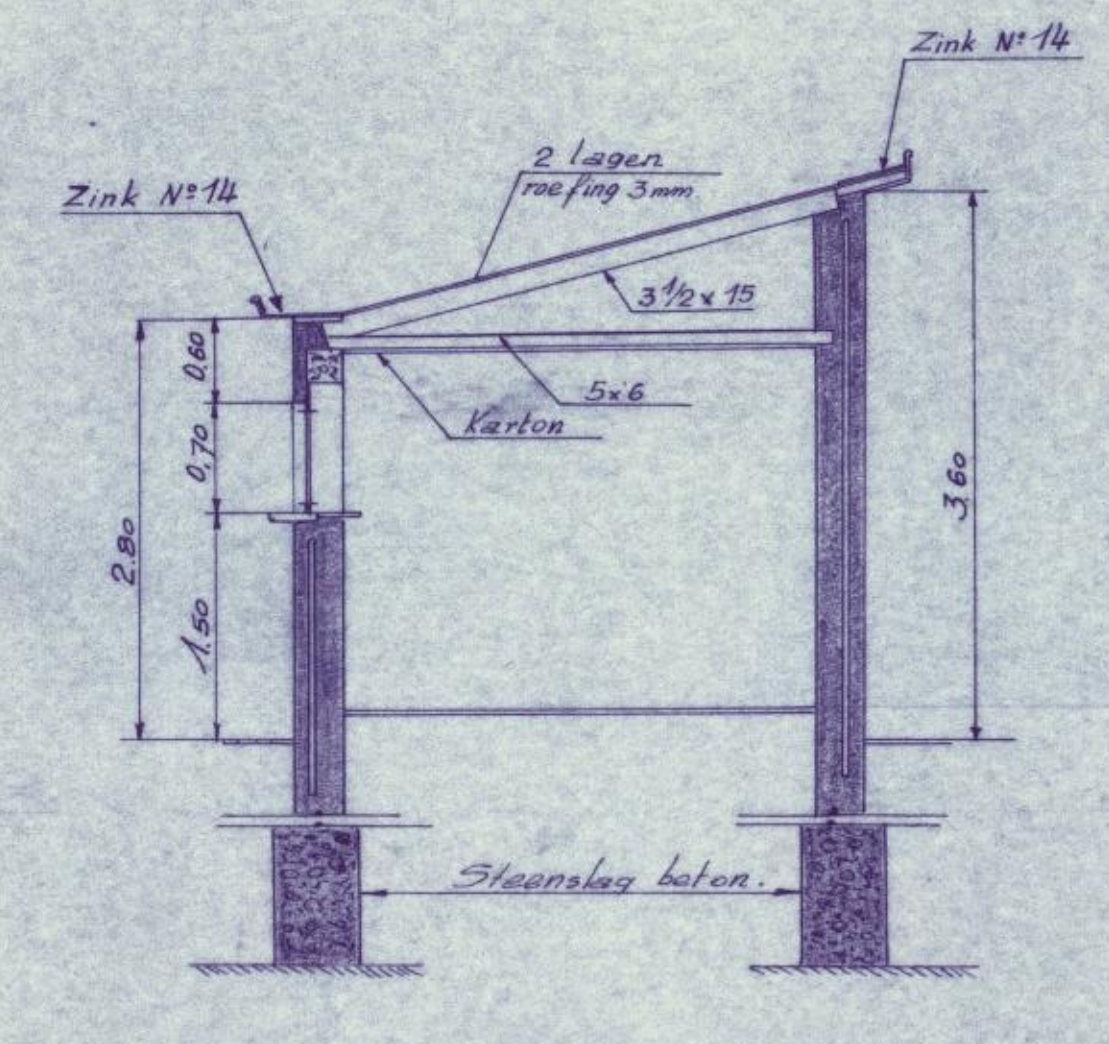
DOORSNEDE C. D.
