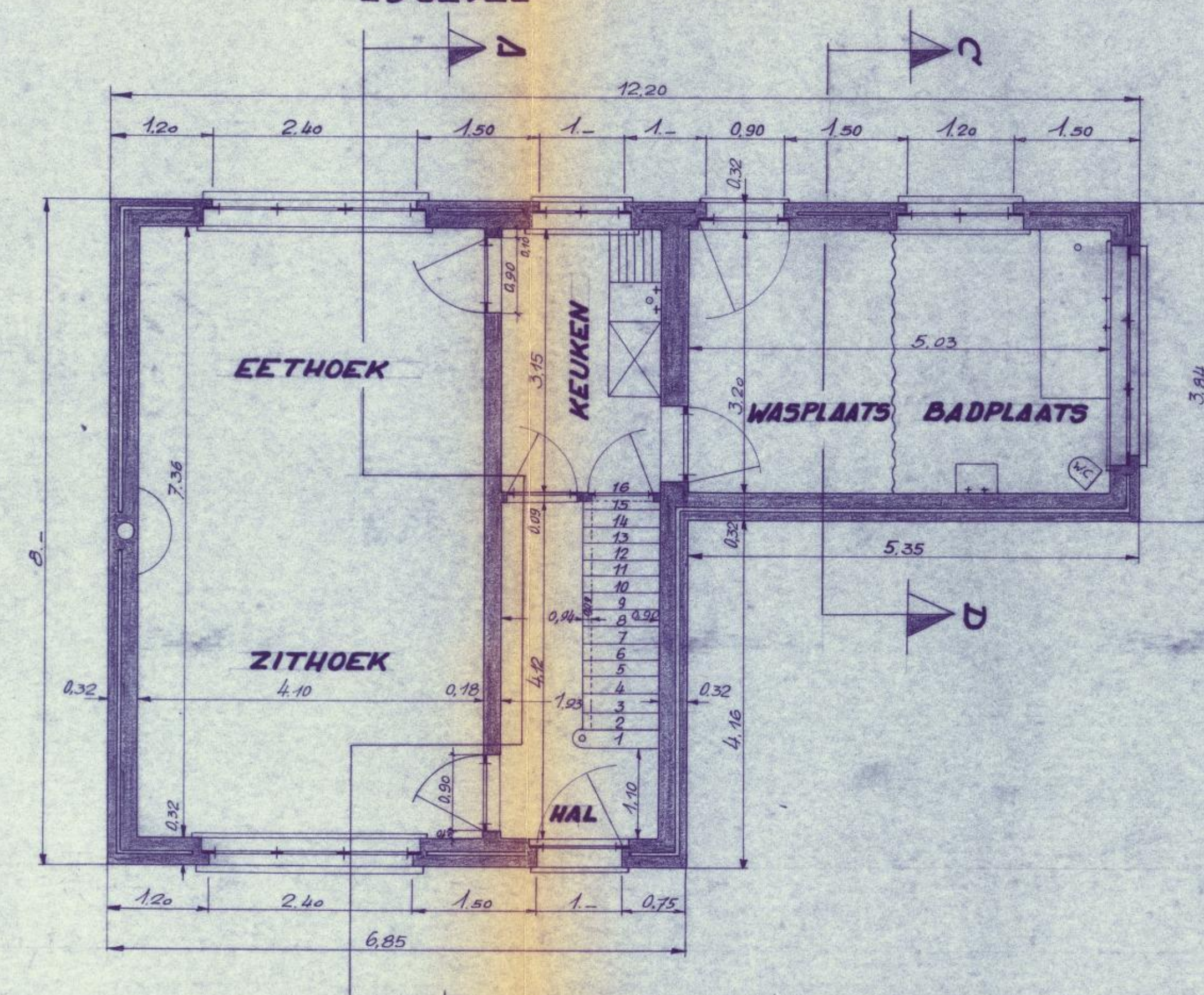
GELUKVLOERS.
