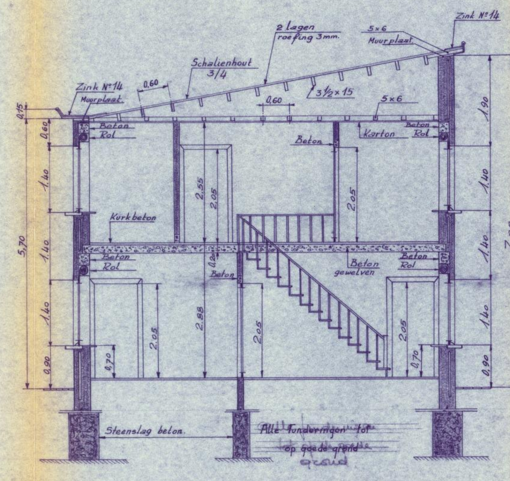
DOORSNEDE A. B.
